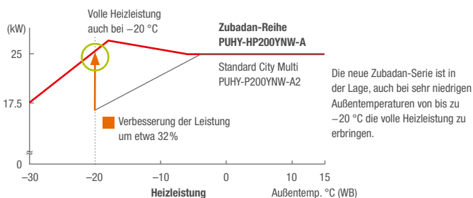
Stabile Heizleistung auch bei -20\text{ }^{\circ}\text{C} (für Baugröße HP200)
