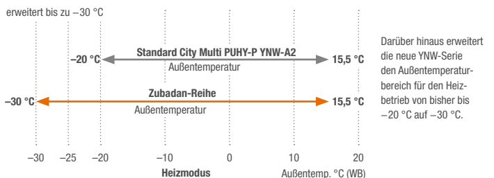
Erweiterter Heizbetrieb bei bis zu -30\text{ }^{\circ}\text{C}
